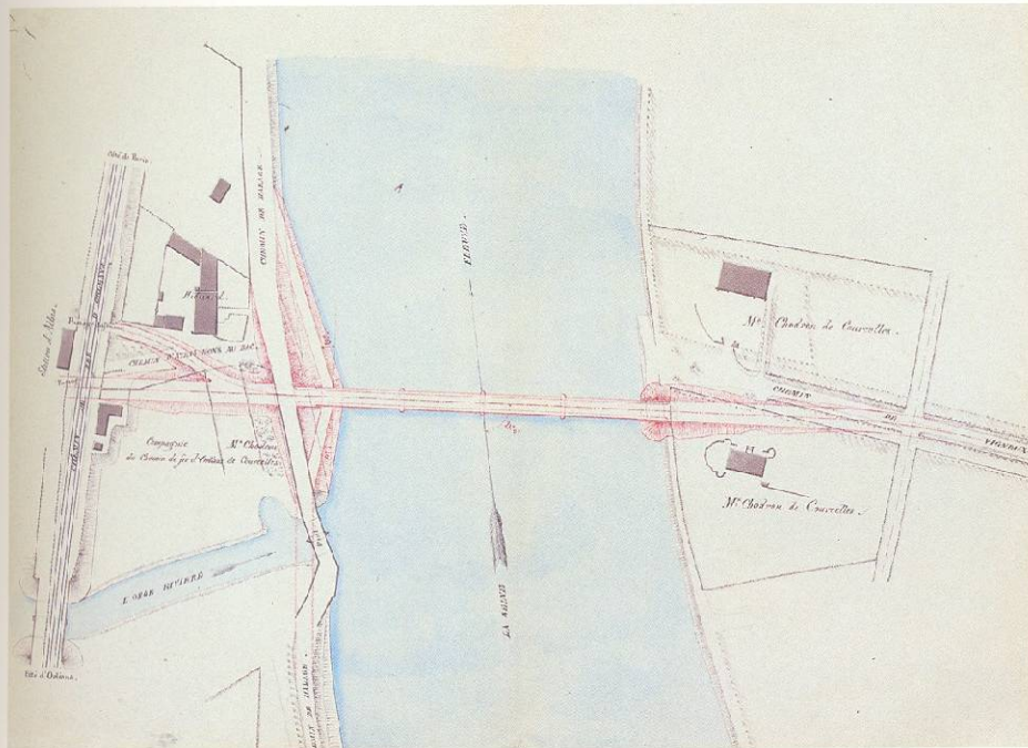
Projet de pont sur la Seine entre Athis-Mons et Vigneux (A.D. Essonne, 2 S 176)
